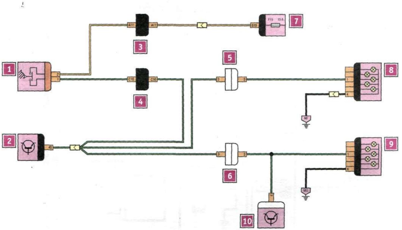
Схема 13. Фонари заднего хода: 1 - выключатель света заднего хода; 2 - блок управления электрооборудованием кузова; 3 - разъем R212; 4 - разъем R212; 5 - разъем R296; 6 - разъем R296; 7 - предохранитель (блок предохранителей и реле в салоне); 8 - правый задний фонарь; 9 - левый задний фонарь; 10 - ЭБУ системы парковки
