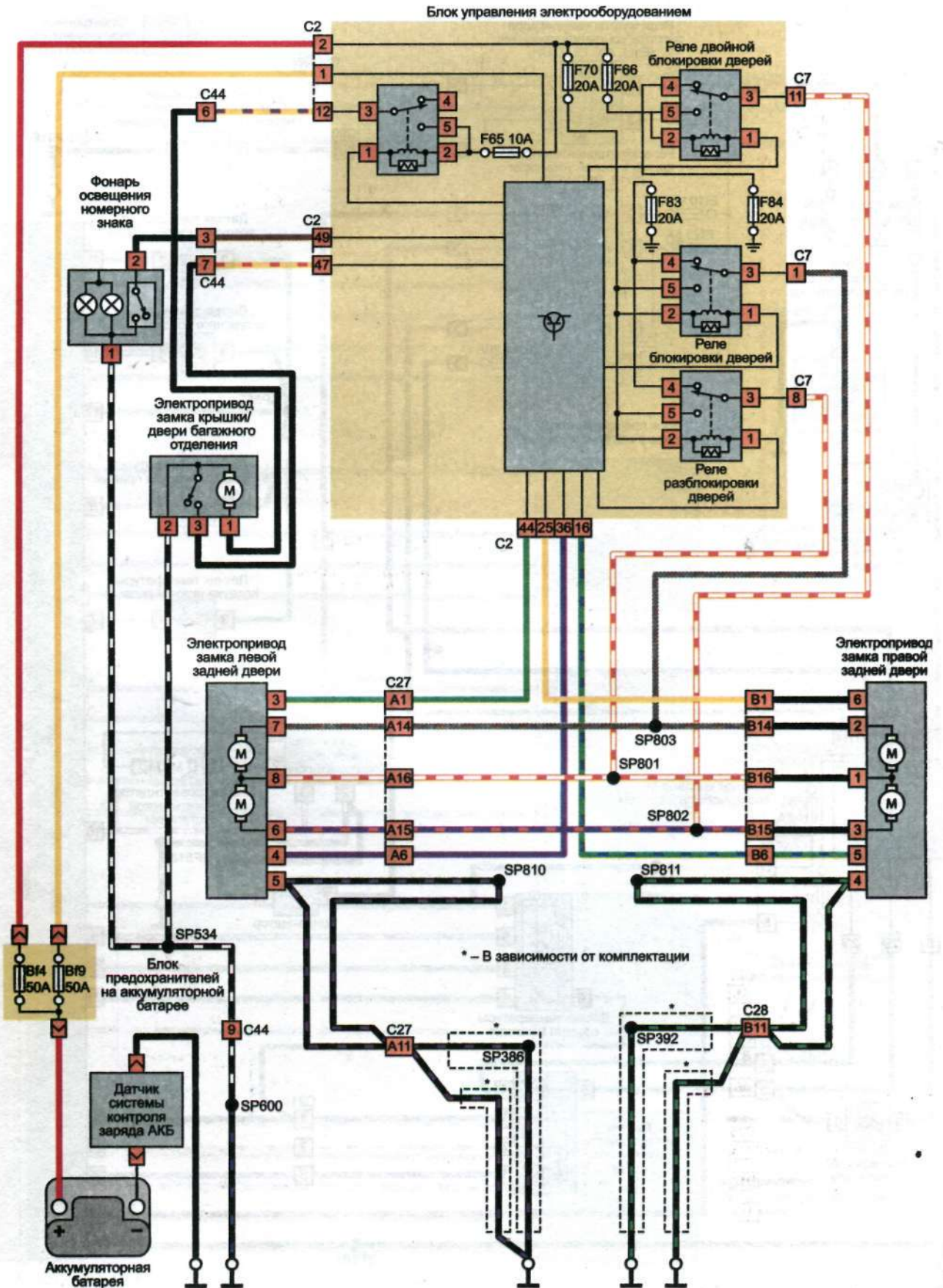
Схема 16.2 Система блокировки дверей
