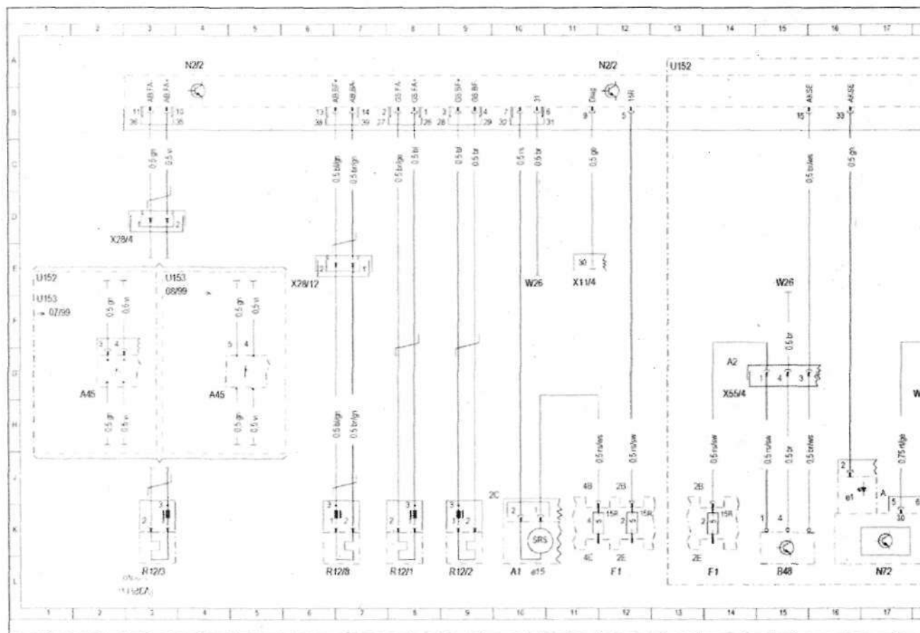
Электрическая схема подушек безопасности на ТИПЕ 202 с 01.06.1998
