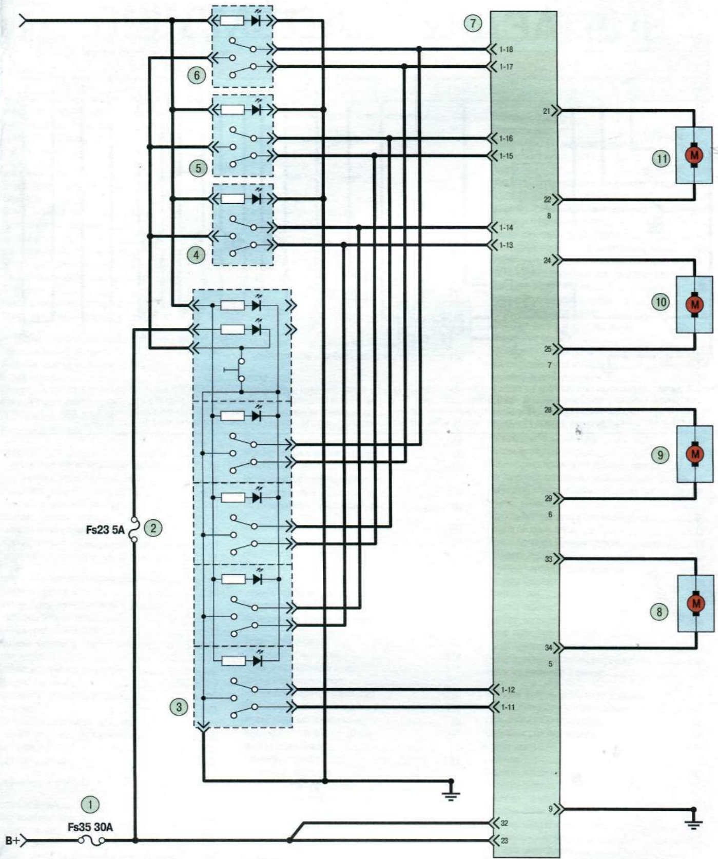
Схема 7. Электрические стеклоподъемники: 1 – предохранитель стеклоподъемников в монтажном блоке, расположенном в салоне; 2 – предохранитель; 3 – центральный блок управления электростеклоподъемниками; 4 – клавиша управления электростеклоподъемником правой передней двери; 5 – клавиша управления электростеклоподъемником правой задней двери; 6 – клавиша управления электростеклоподъемником левой задней двери; 7 – блок управления кузовным электрооборудованием; 8 – моторредуктор стеклоподъемника левой передней двери; 9 – моторредуктор стеклоподъемника правой передней двери; 10 – моторредуктор стеклоподъемника левой задней двери; 11 – моторредуктор стеклоподъемника правой задней двери
