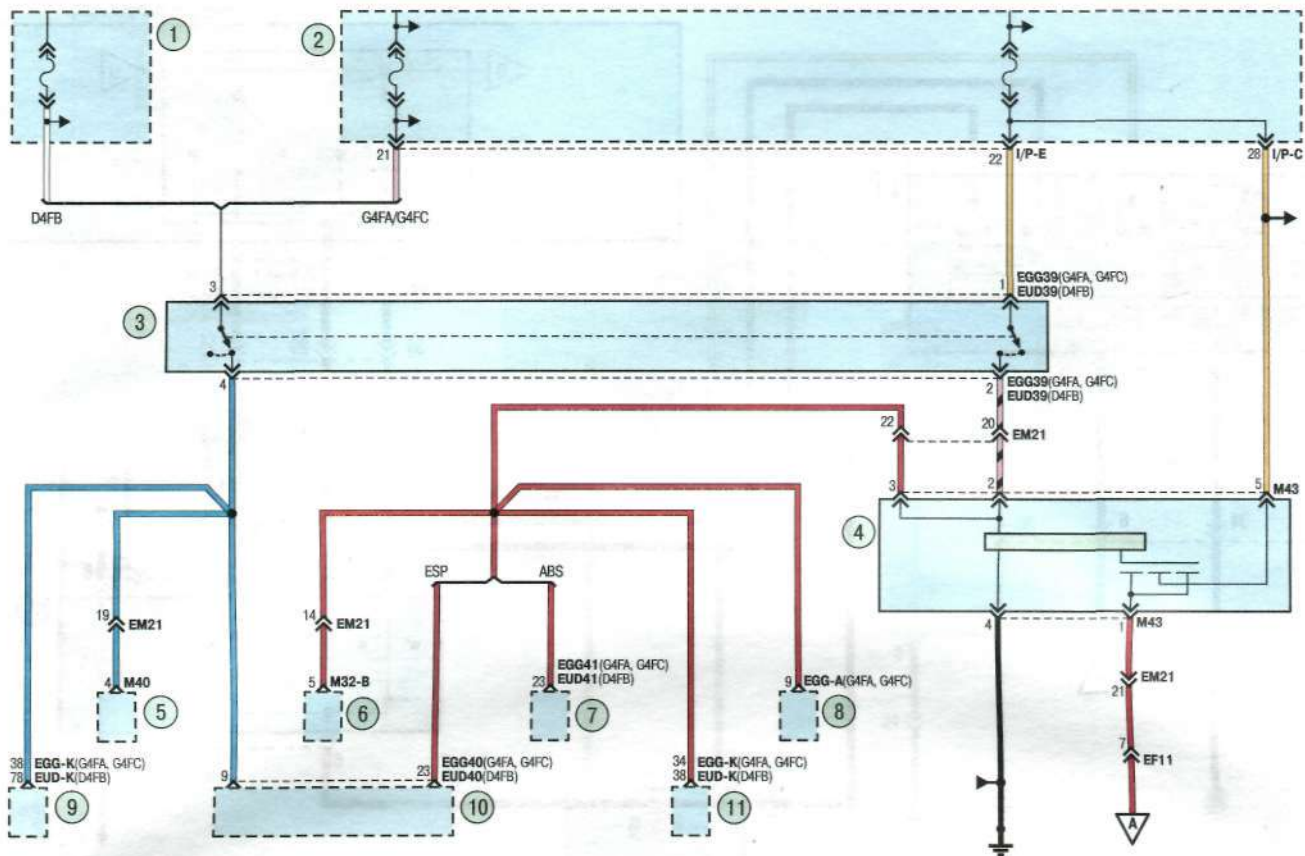
Схема 16. Система ABS: 1 – монтажный блок в моторном отсеке; 2 – монтажный блок в салоне автомобиля; 3 – выключатель стоп-сигнала; 4 – реле ламп стоп-сигнала; 5 – модуль контроля включения блокировки руля; 6 – электронный ключ зажигания; 7 – гидроэлектронный модуль ABS; 8 – модуль управления трансмиссией; 9, 11 – электронный блок управления двигателем; 10 – модуль управления системой ESP
