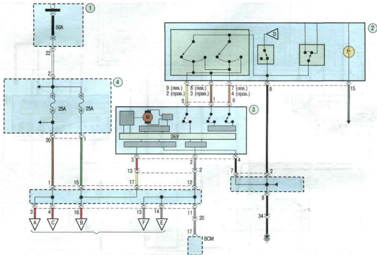
Схема 17. Электростеклоподъемник двери водителя (с интеллектуальным модулем привода): 1 – блок реле и предохранителей в моторном отсеке; 2 – блок управления стеклоподъемниками, зеркалами заднего вида и блокировкой замков дверей (с интеллектуальным модулем привода стеклоподъемников); 3 – интеллектуальный модуль привода стеклоподъемника двери водителя; 4 – блок реле и предохранителей в салоне автомобиля
