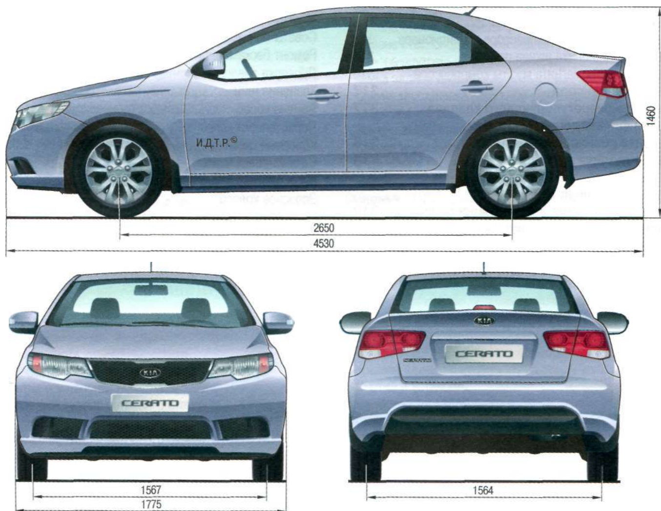
Рис. 1.1. Габаритные размеры автомобиля Kia Cerato
