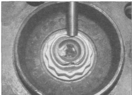
Рис. 3.28. Окончательно затянув ступичную гайку, вдавите буртик в канавки вала
