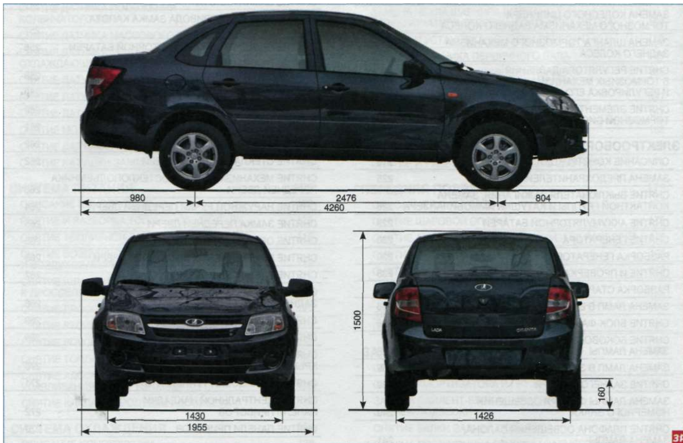
Габаритные размеры автомобиля
