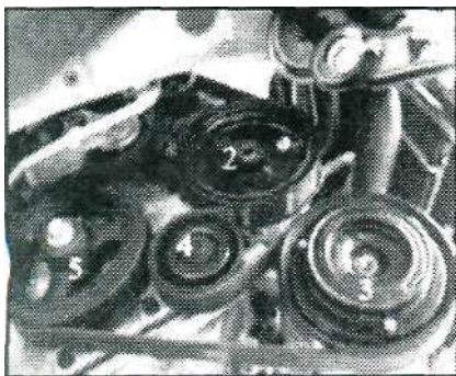
Рис. 4.2.1. Расположение приводного ремня:
