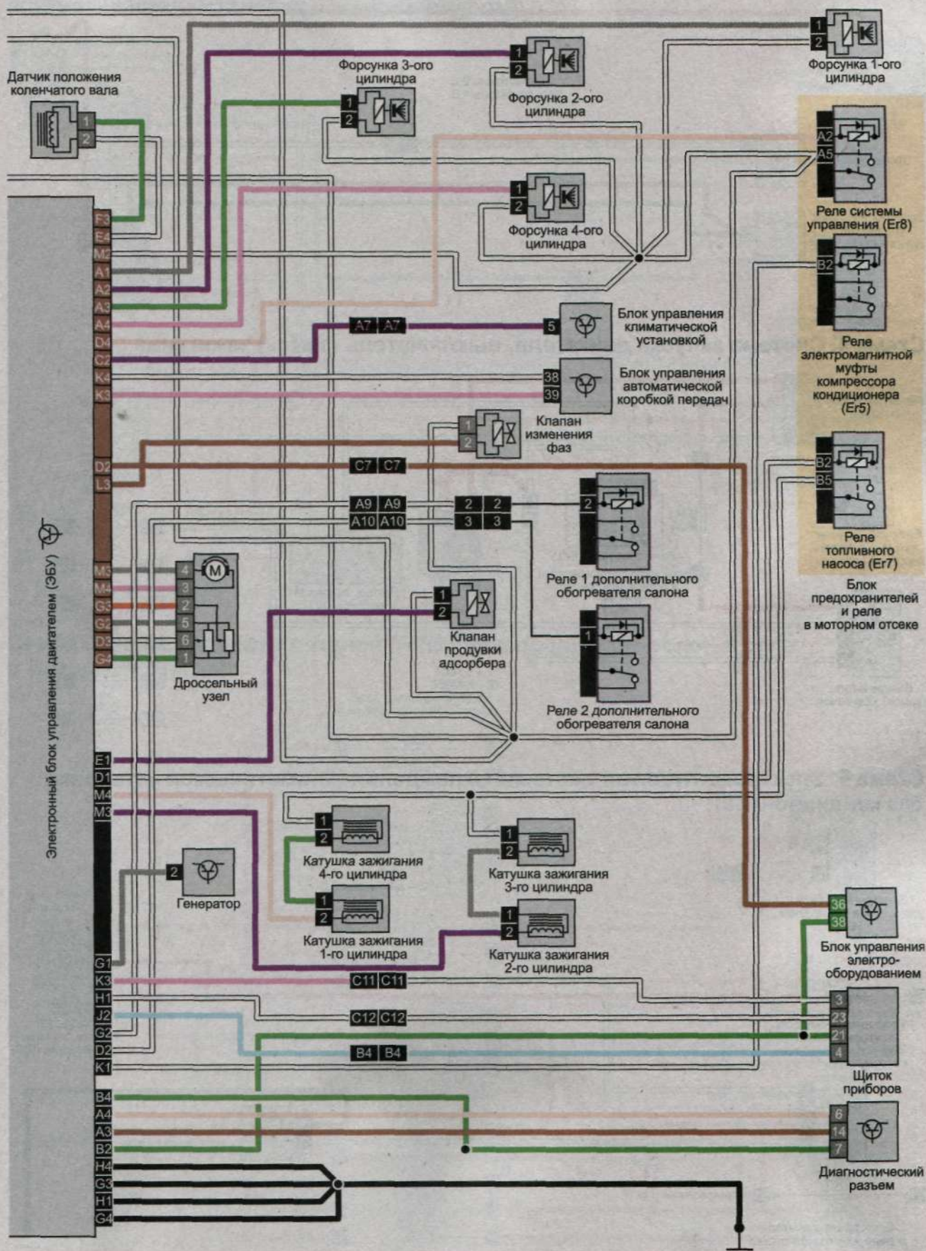
Схема 2.2 Система управления двигателем 2,0 (окончание)
