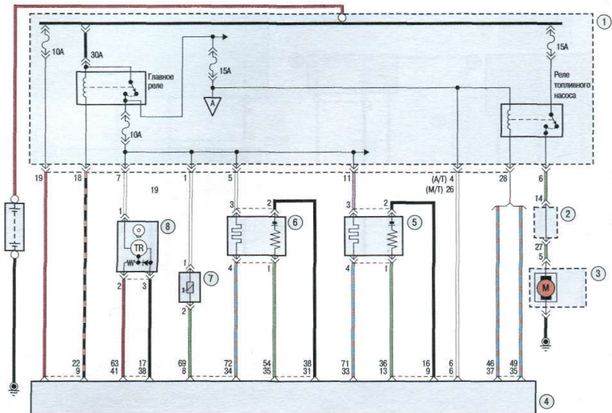
Схема 1а. Система управления двигателем: 1 – блок реле и предохранителей в моторном отсеке; 2 – блок реле и предохранителей в салоне автомобиля; 3 – топливный модуль; 4 – электронный блок управления двигателем; 5 – диагностический датчик концентрации кислорода; 6 – управляющий датчик концентрации кислорода; 7 – электромагнитный клапан системы улавливания паров топлива; 8 – датчик положения распределительного вала
