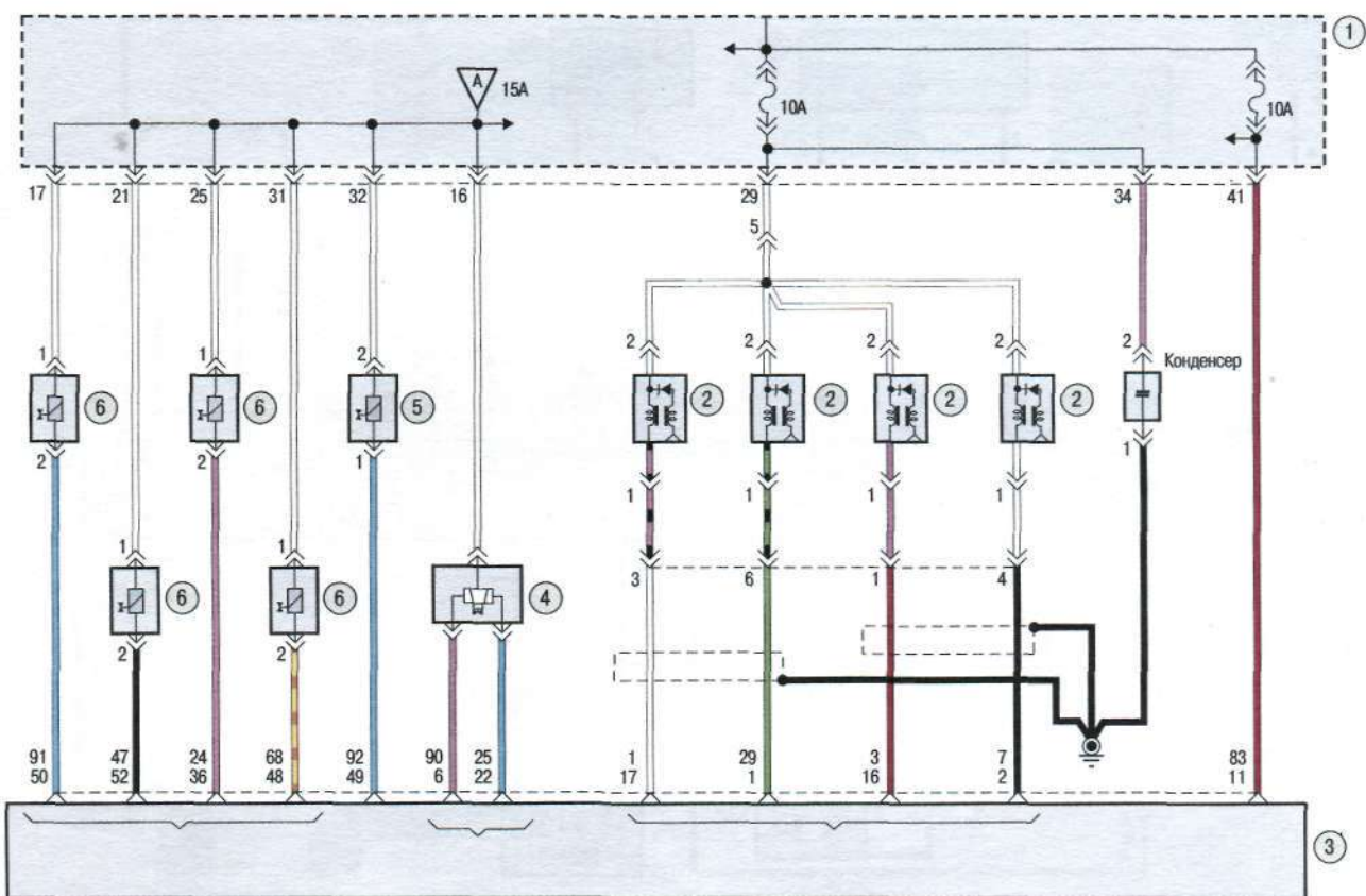
Схема 1б. Система управления двигателем: 1 – блок реле и предохранителей в моторном отсеке; 2 – катушка зажигания; 3 – электронный блок управления двигателем; 4 – регулятор холостого хода; 5 – электромагнитный клапан изменения фаз в системе газораспределения; 6 – форсунка
