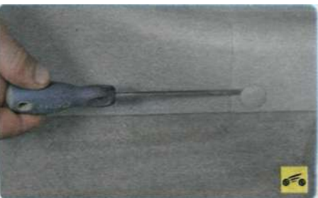
3. Для снятия передней облицовки порога подденьте отверткой...
