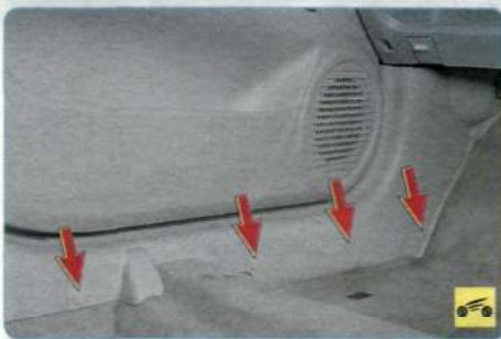
4. ...и извлеките пистоны крепления облицовки.
