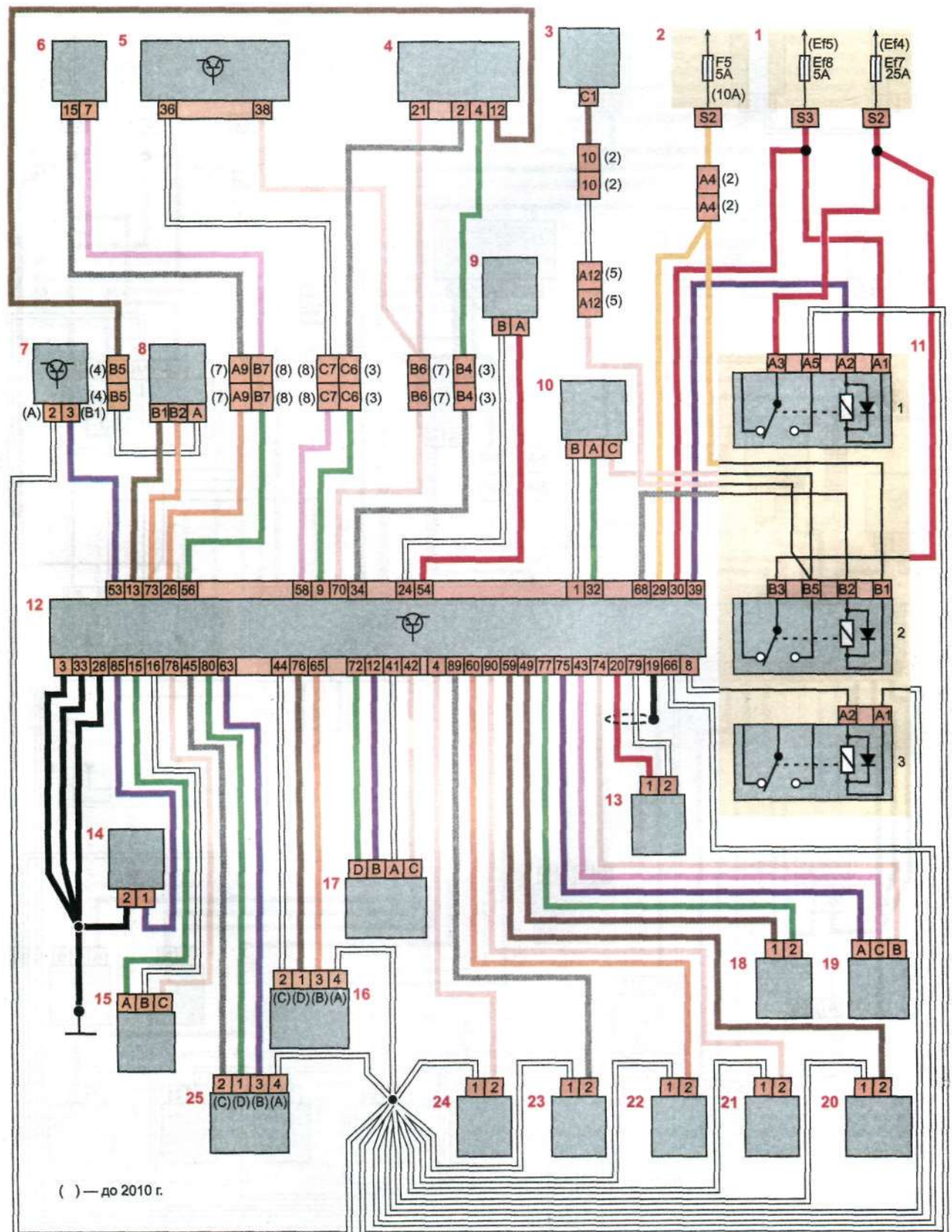
Схема 4. Система управления 8-клапанного двигателя
