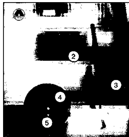
2. Стяжная часть 3. Крепежная лента 4. Крючок для предохранительной сетки 5. Крепежная проушина
