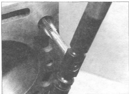
Рис. 11.8. Метчиком прогоните резьбы отверстий блока
